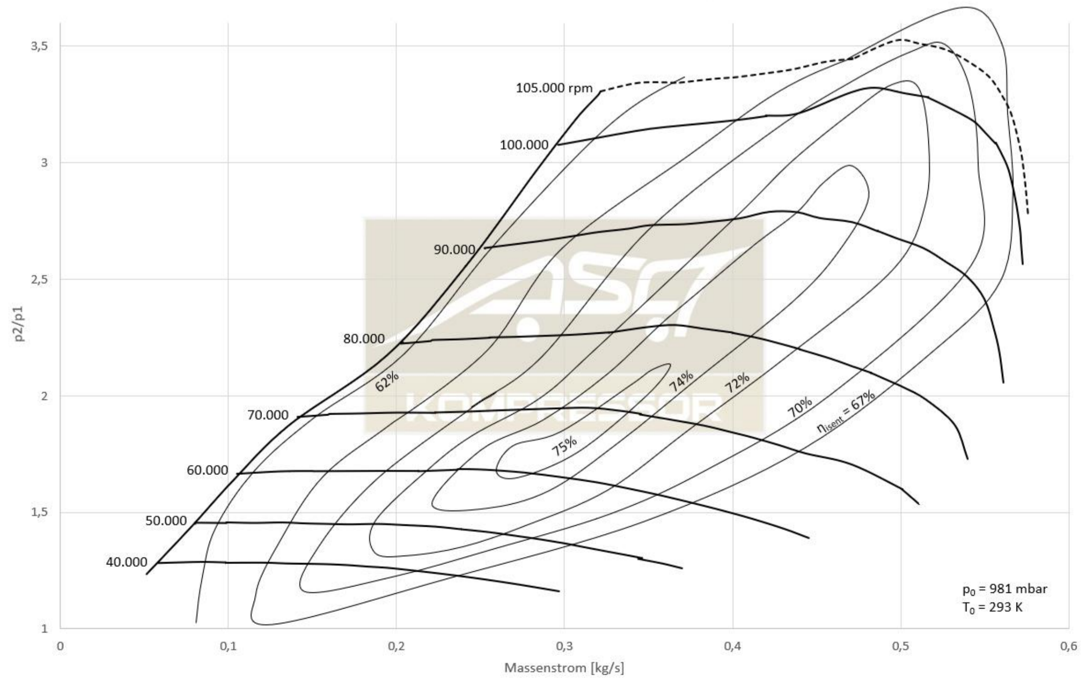
Verdichterkennfeld flow chart T1-520
