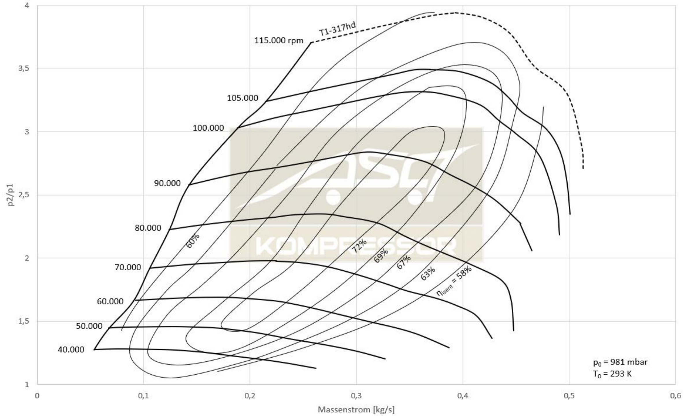
Verdichterkennfeld flow chart T1-317 (hd)
