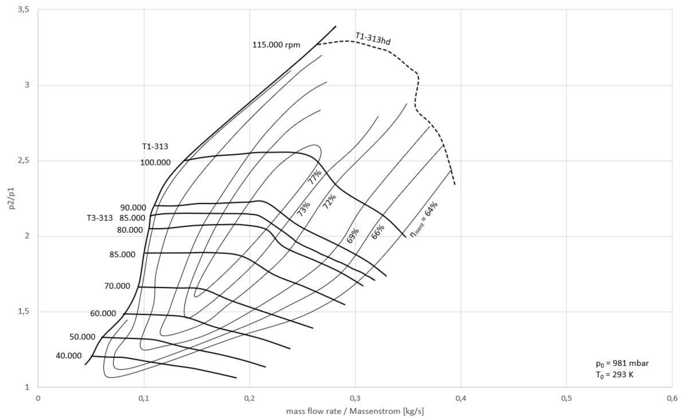
Verdichterkennfeld flow chart T3-313
