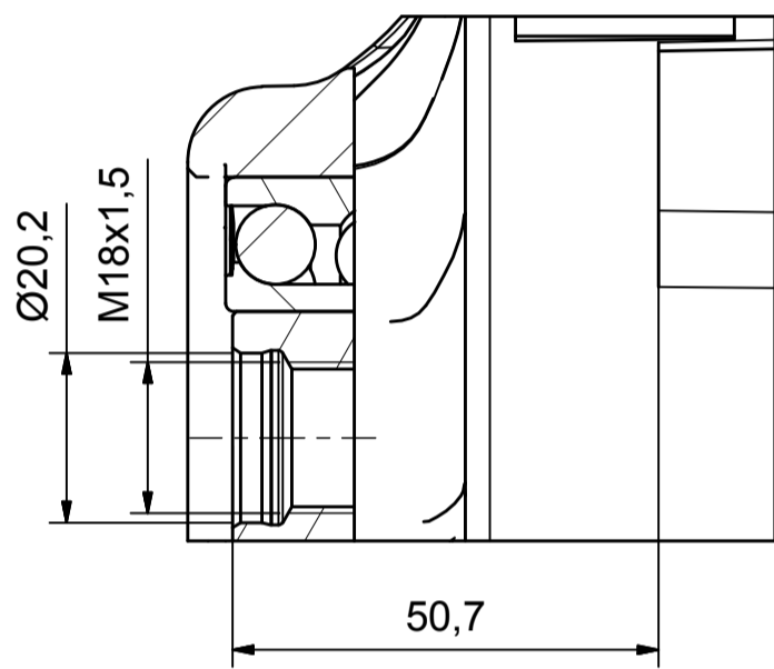
A (2 : 1) Antrieb
