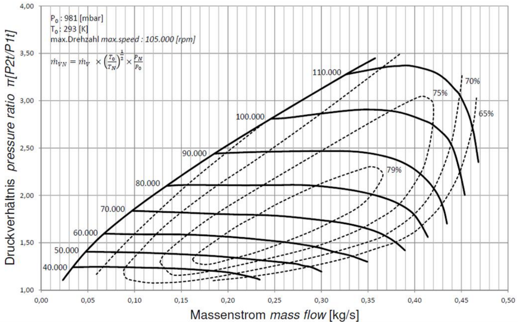
Verdichterkennfeld flow chart T1-316 (3470)
