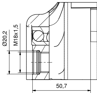
A ( 2 : 1 ) Antrieb drive
